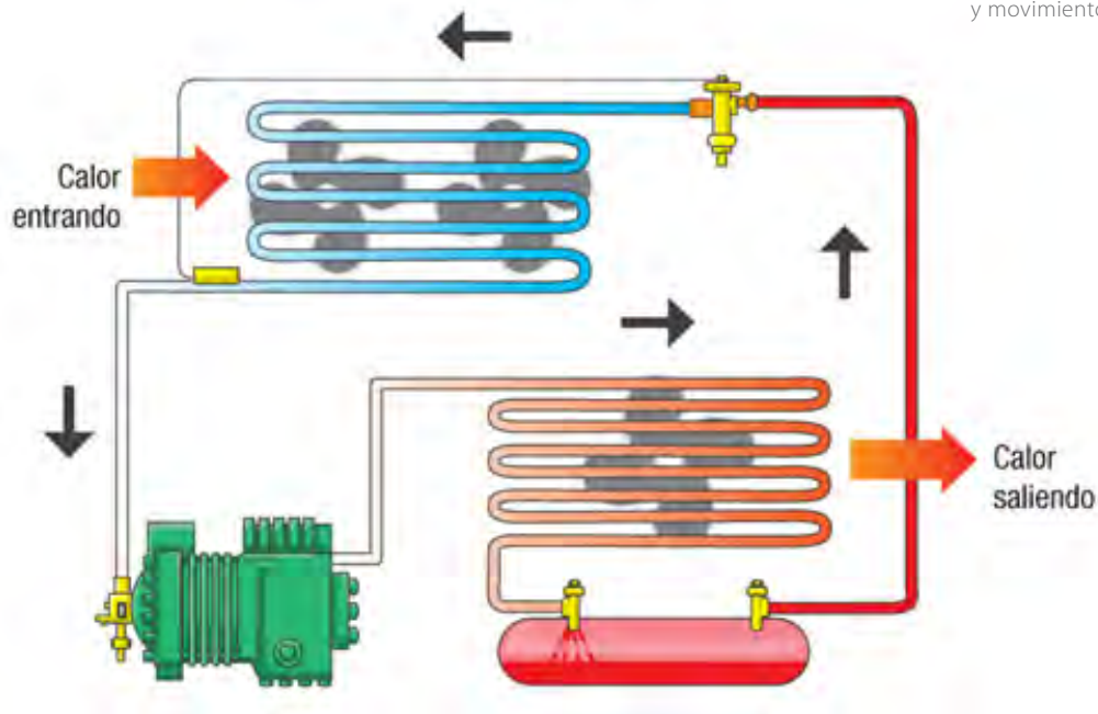
Figura 2: Ciclo de refrigeración y movimiento de energía.
